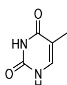
Thymin (DNA)
