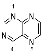
Pteridin
