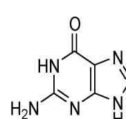
Guanin (DNA)
