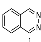
Phthalazin
