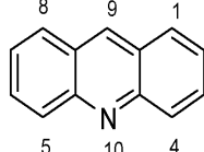
Acridin
