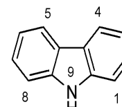
Carbazol
