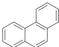
Phenanthren farblos
