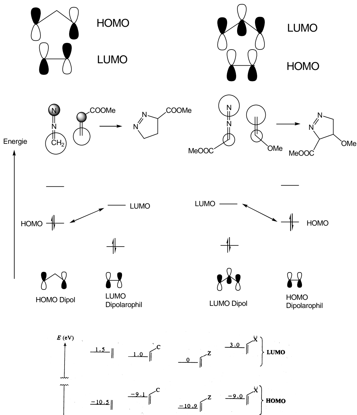
Energien der Grenzorbitale von Dienophilen. C = Vinyl oder Phenyl; Z = CHO, CN, NO 2 etc; X = CH 3 O, (CH 3 ) 2 N, CH 3 etc. Die Energien (in eV) sind typische Werte für jede Klasse von Dienophilen (1 eV = 96.5 kJ = 23 kcal).
