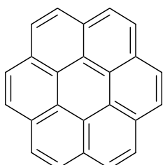
Coronen
