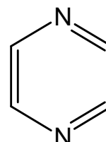
Pyrazin pKs 0,5
