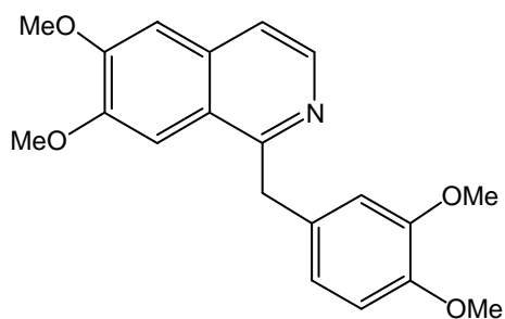
Papaverin:
