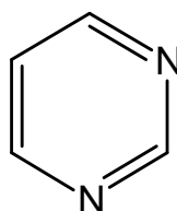
Pyrimidin pKs 1,3
