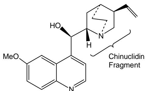
Chinin:
