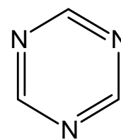
1,3,5-Triazin
