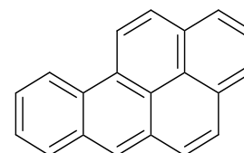
Benzo[a]pyren
