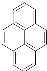
Pyren
