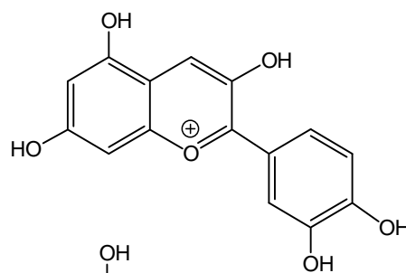
Cyanidin (blau)
