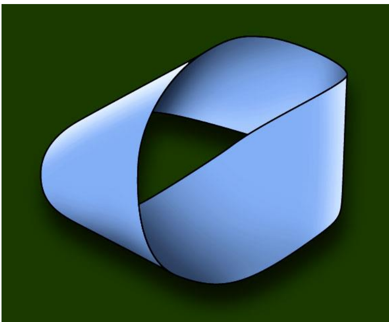
Möbiusband (chiral)
