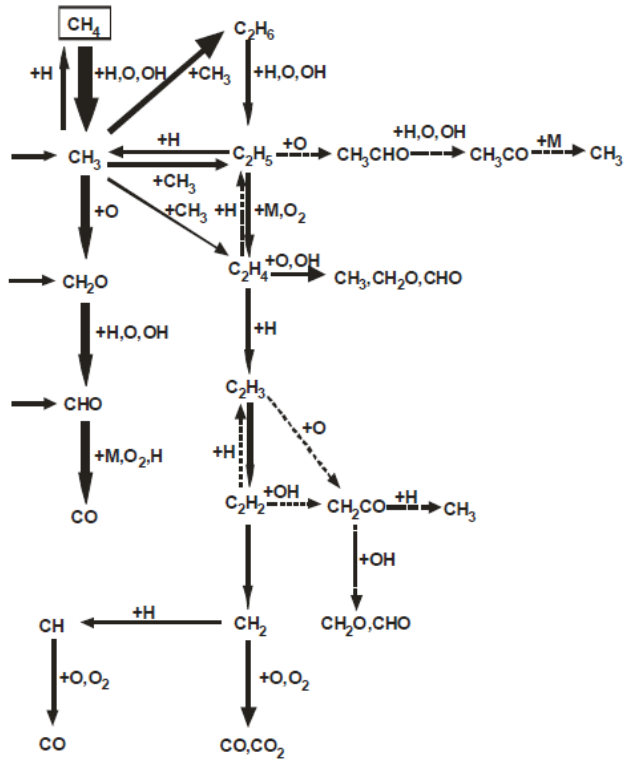
Bild 4-1: Integrale Reaktionsflussanalyse in einer vorgemischten stöchiometrischen Methanflamme (Warnatz 1984)
