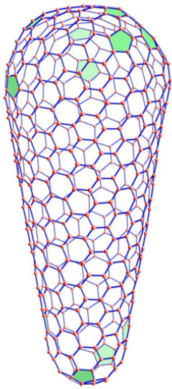
Symmetrie eines konischen Viruskapsids (HIV-1)
