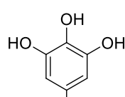
Gallussäure
