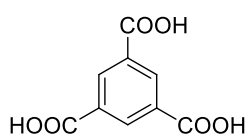
Trimesinsäure
