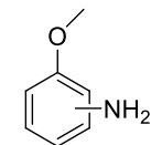
o,m,p-Anisidin
