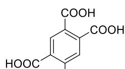
Pyromellitsäure
